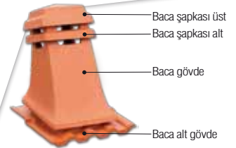
Baca (Ebat 47X43 cm) Dört kiremit büyüklüğünde tek parçadır. Dekoratif hazır baca seti gövdesi ve şapkası uygulama kolaylığı sağlar
